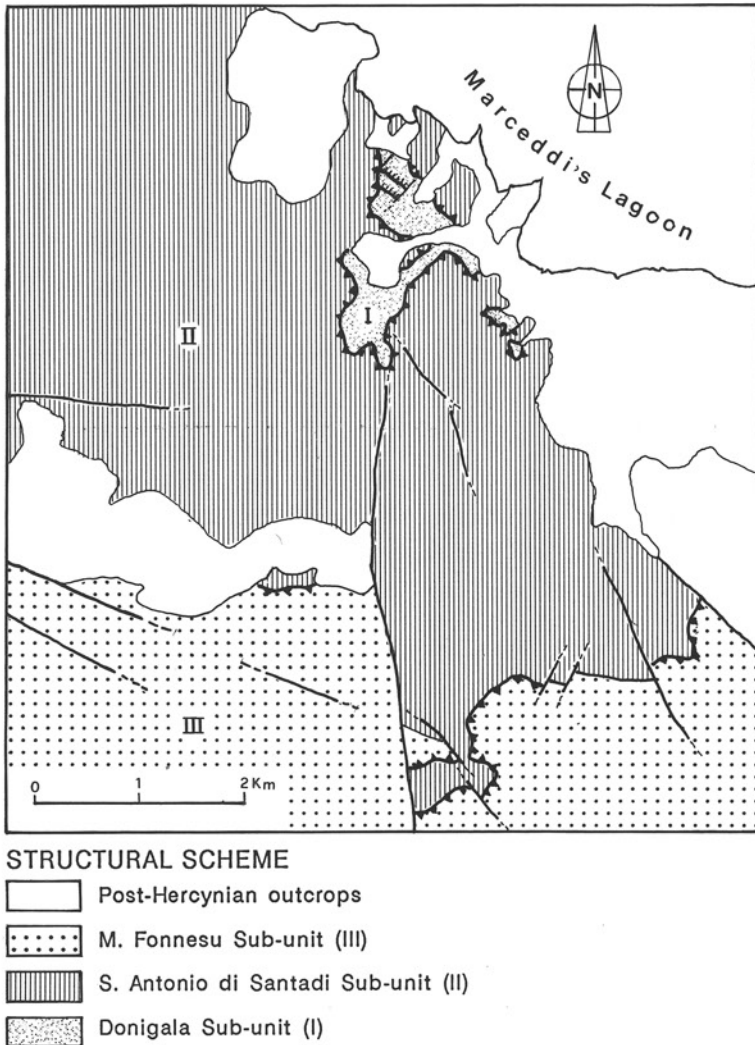
Fig. 2 - Structural scheme of the S. Antonio di Santadi area.
