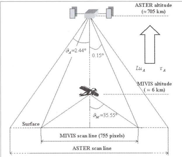
Figura 1 - Caratteristiche geometriche dell'ASTER e del MIVIS.
