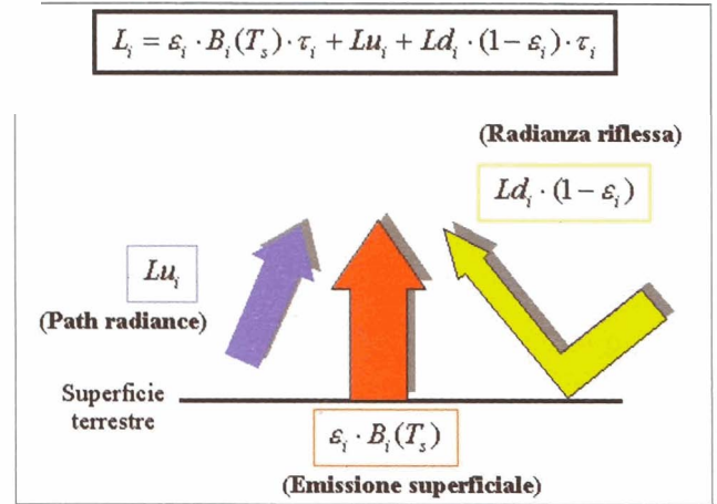
Figura 2 - Equazione del trasferimento radiativo nel TIR.
