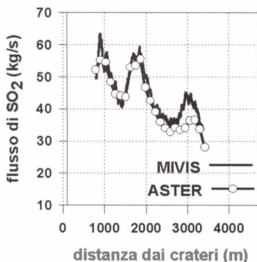
Figura 6 - 12 giugno 1997 - Andamento del flusso di \text{SO}_2 lungo l'asse del plume calcolato dall'immagine ASTER simulata e ottenuto direttamente dalle immagini MIVIS.
